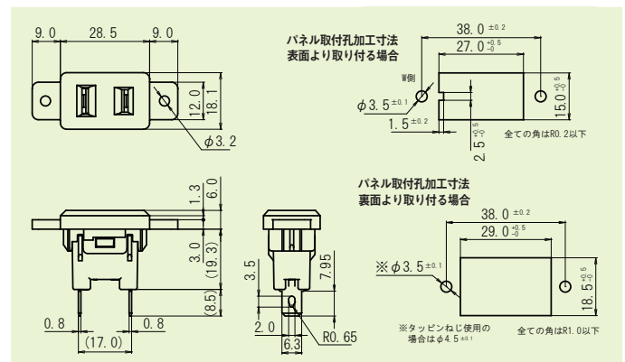
S-250-W S-250-B 仕様
