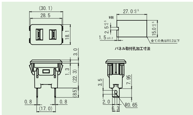
S-200-W S-200-B 仕様
