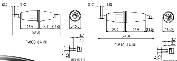
端子部寸法
